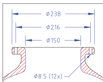
DÉTAIL BRIDE DE 6"
