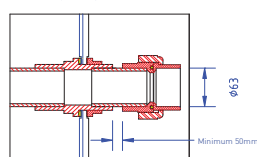
DÉTAIL ORIFICE LATÉRAL
