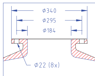
DÉTAIL BRIDE DE DN200
