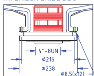
DÉTAIL SUPÉRIEUR/ INFÉRIEUR BRIDE DE 6"
