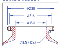
DÉTAIL BRIDE DE 6"
