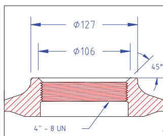
Détail Filetage 4"
