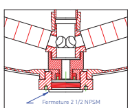
DÉTAIL FILETAGE DE 4"
