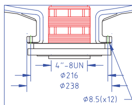
DÉTAIL BRIDE INFÉRIEURE DE 6" 3E
